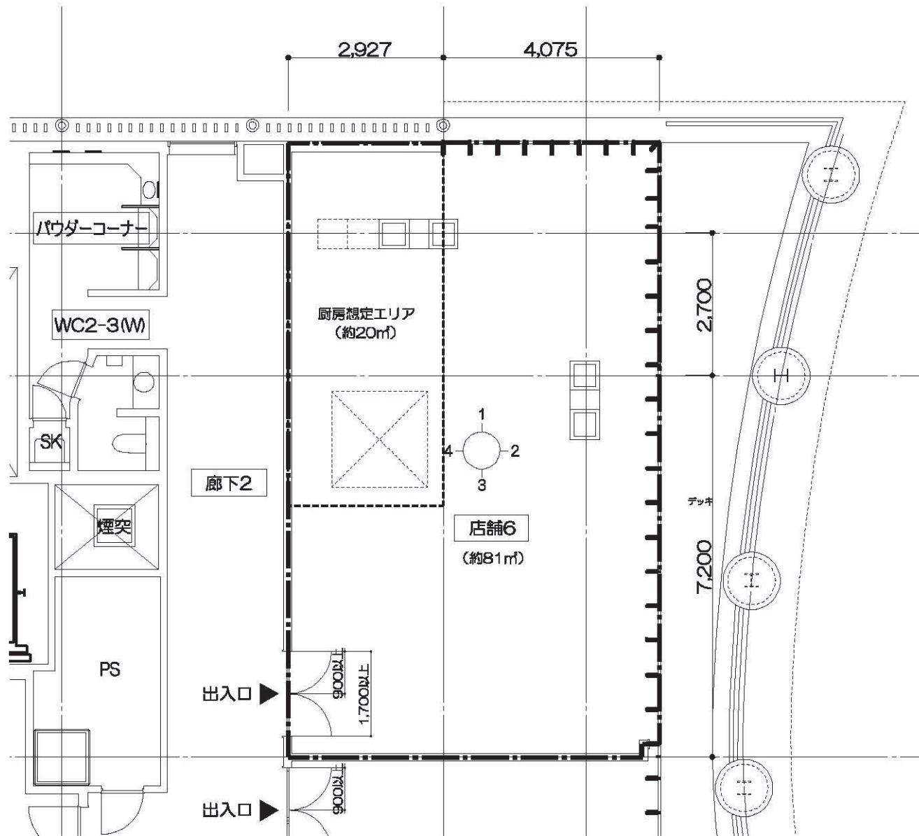
平面図 S=1:100
